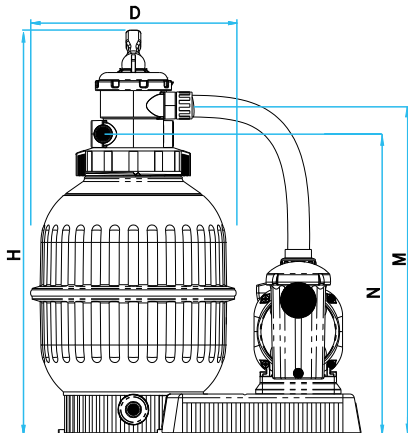
Monoblocco Top Top-mount monobloc
