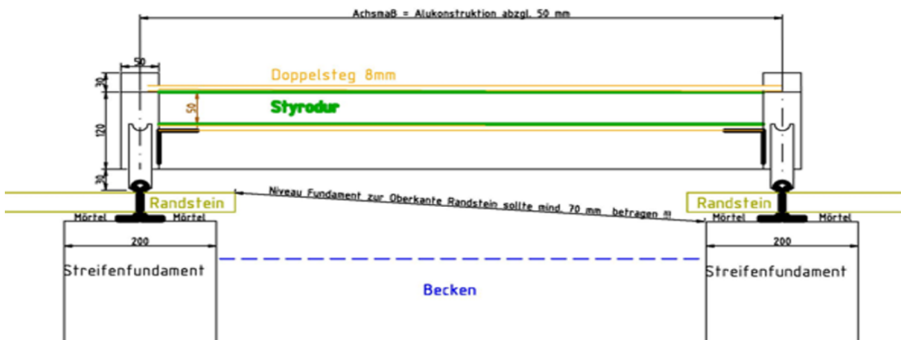
Beispiel beidseitig versenkte Laufschiene am 120er Kastenprofil Spann bis 5000 mm
