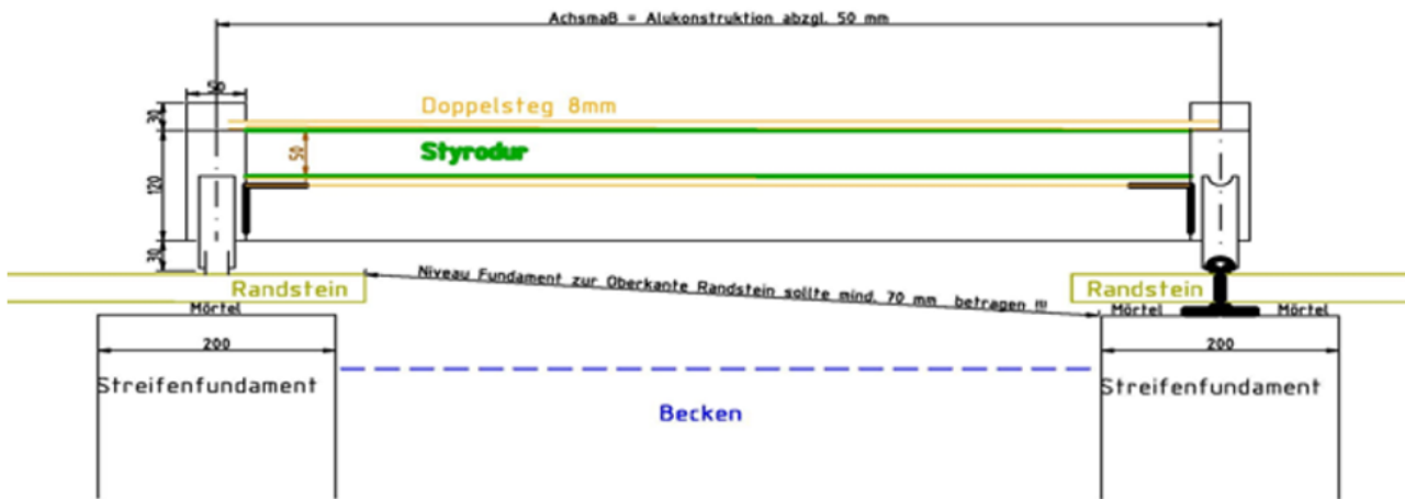
Beispiel einseitig versenkte Laufschiene am 120er Kastenprofil Spann bis 5000 mm
